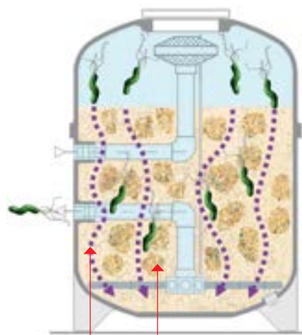
Zandfilter Zuurstofloze gebieden in het filterbed Kanaalvorming in het filterbed
